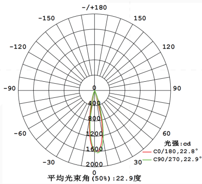
配光曲线图
