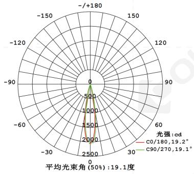
配光曲线图
